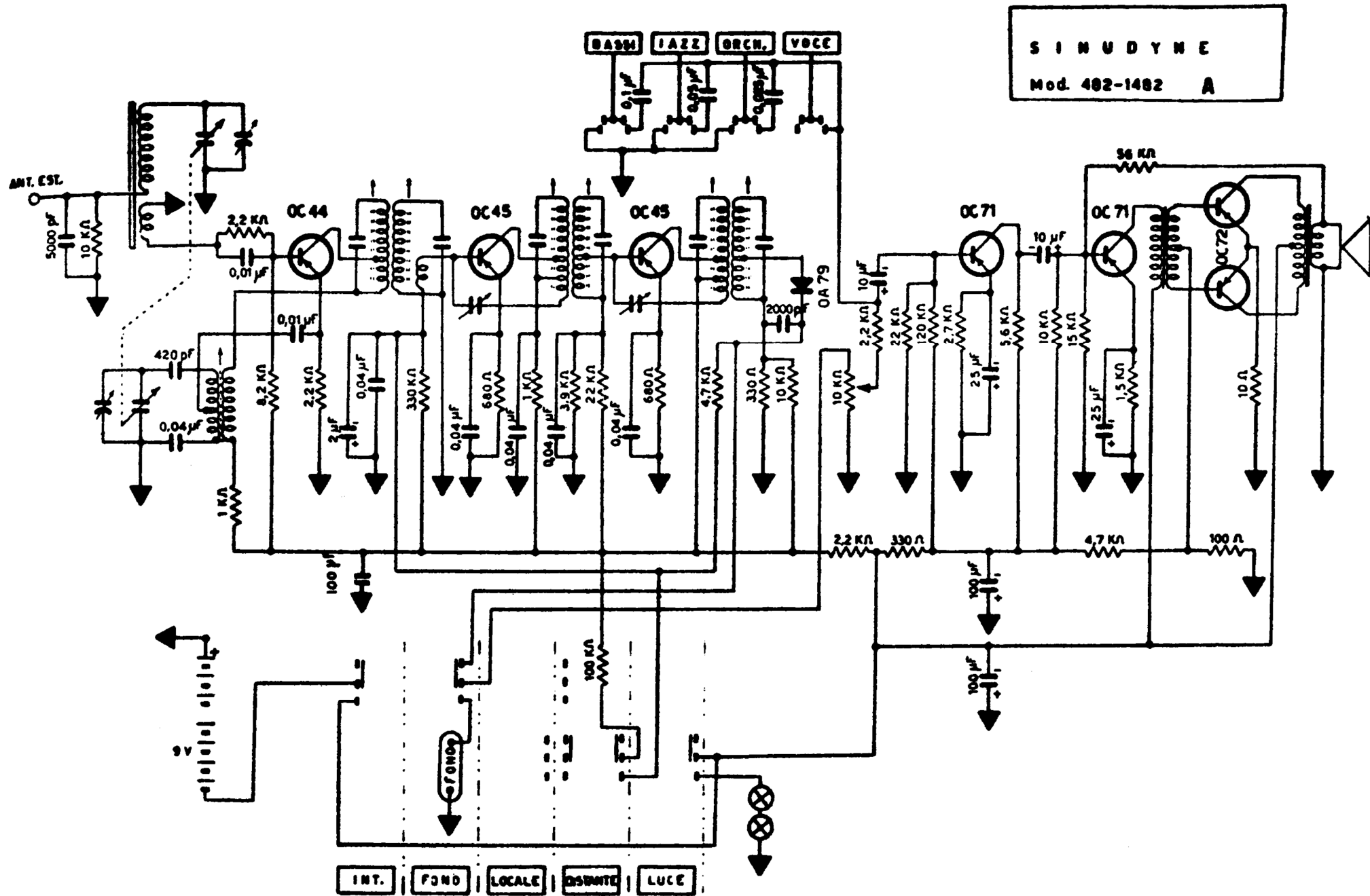
SINUDYNE - Modd. 482 e 1482. Apparecchi portatili a sette transistor, con gamma onde medie. L'apparecchio è provvisto di presa fono, e di commutatore locale-distante, con commutazione a tasti. È pure provvisto di registro di tonalità a quattro tasti. Media frequenza AM a 468 kc/s, media frequenza FM a 10,7 Mc/s.
